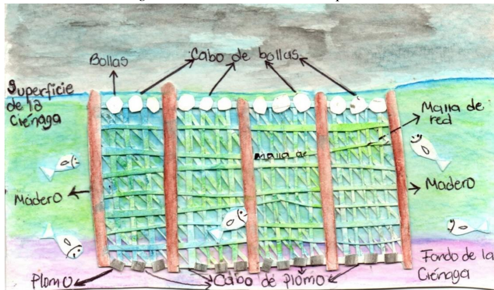
Figura 4. Trasmallo estacionario o para'ó.
