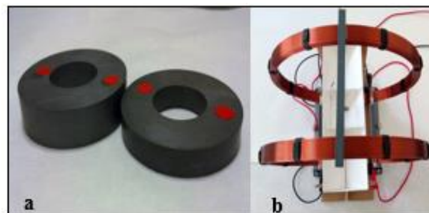
Figura 1a. Los imanes generan campos magnéticos estacionarios. Imán de 250 mT (izquierda) e imán de 125 mT (derecha). Fuente: Álvarez, J. 1b. Las bobinas generan campos magnéticos alternos. Bobina de Helmholtz. Fuente: Álvarez, J.
