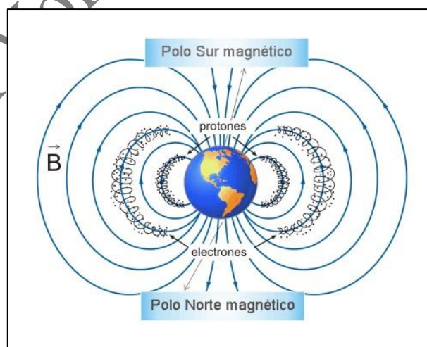
Figura 2. Líneas de campo magnético de la Tierra. Las partículas cargadas (protones y electrones) que provienen de las radiaciones solares se quedan atrapadas en las líneas de campo formando los cinturones de Van Allen. Fuente: Tipler y Mosca (2008).
