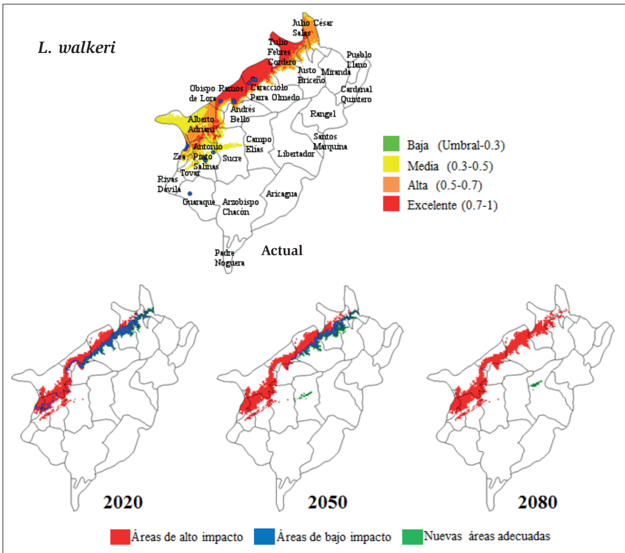
Figura 5. Mapa de distribución actual y bajo escenarios de cambio climático de L. walkeri para los años 2020, 2050 y 2080 en el estado Mérida Venezuela. La predicción futura se realizó con el modelo matemático Hadcm3 en el escenario pesimista A2, utilizando las capas de 19 variables bioclimáticas derivadas de temperatura y precipitación.
