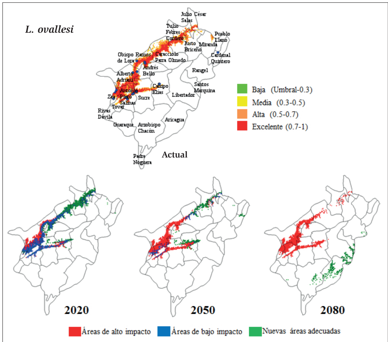
Figura 4. Mapa de distribución actual y bajo escenarios de cambio climático de L. ovallesi para los años 2020, 2050 y 2080 en el estado Mérida Venezuela. La predicción futura se realizó con el modelo matemático Hadcm3 en el escenario pesimista A2, utilizando las capas de 19 variables bioclimáticas derivadas de temperatura y precipitación.
