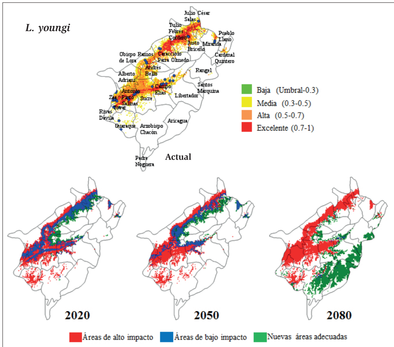
Figura 2. Mapa de distribución actual y bajo escenarios de cambio climático de L. youngi para los años 2020, 2050 y 2080 en el estado Mérida Venezuela. La predicción futura se realizó con el modelo matemático Hadcm3 en el escenario pesimista A2, utilizando las capas de 19 variables bioclimáticas derivadas de temperatura y precipitación.
