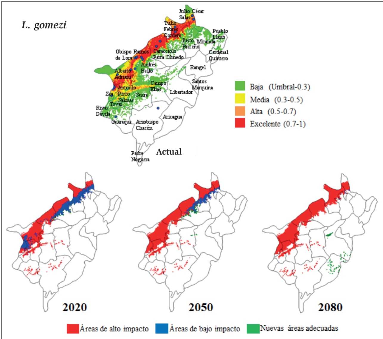
Figura 3. Mapa de distribución actual y bajo escenarios de cambio climático de L. gomezi para los años 2020, 2050 y 2080 en el estado Mérida Venezuela. La predicción futura se realizó con el modelo matemático Hadcm3 en el escenario pesimista A2, utilizando las capas de 19 variables bioclimáticas derivadas de temperatura y precipitación.
